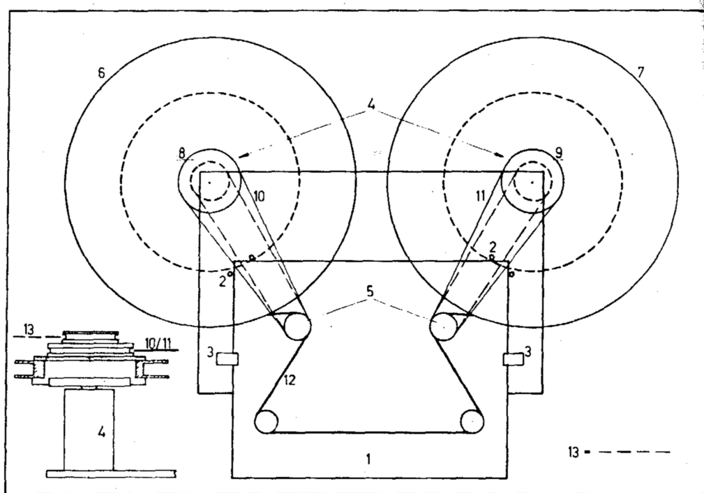
0.3: Abr Large Reel Adaptor
